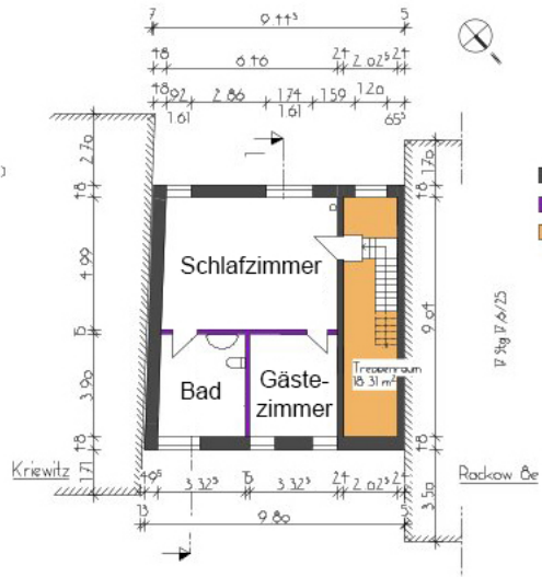
1. Obergeschoß M1.100
